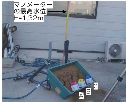
崩壊直前におけるマノメーターの水位
