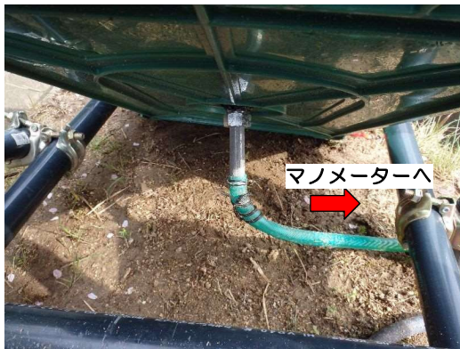
図-3 土槽の裏側から接続したマノメーター
