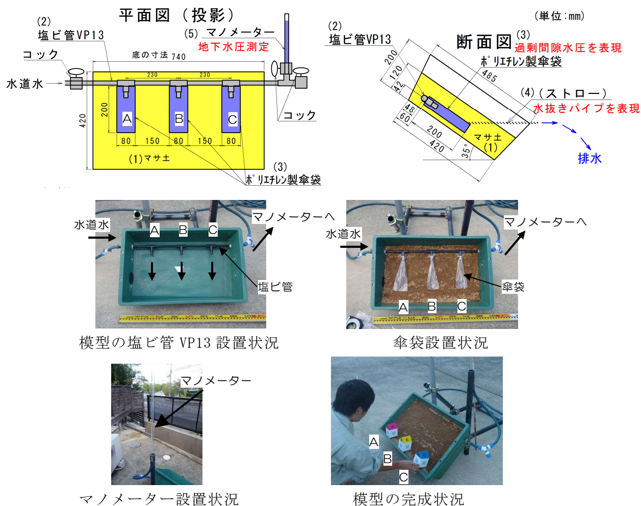
図-8 模型実験装置 (最上部のイラストは模型の模式図)
