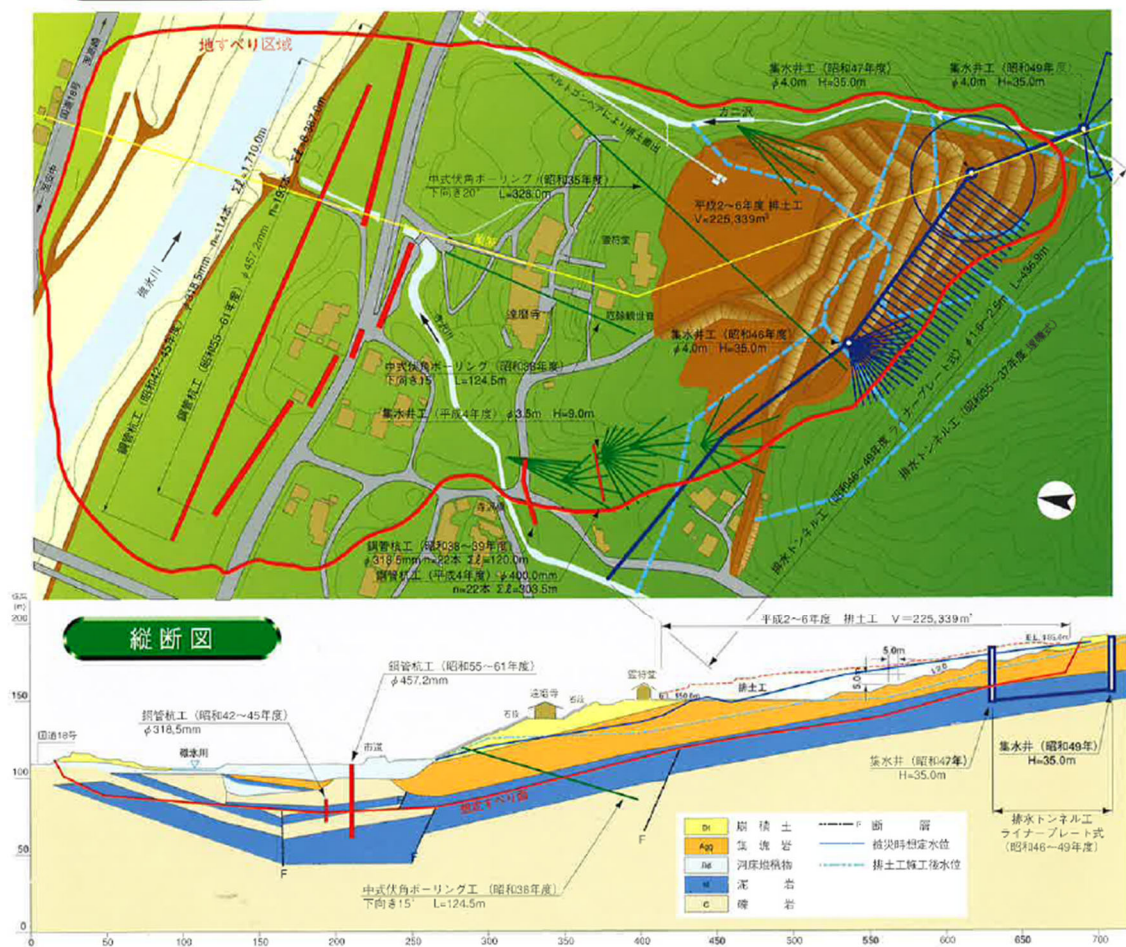
少林山地すべり 概要図
