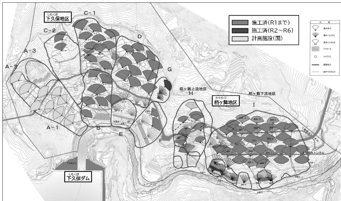
譲原地すべりににおける対策工の概要
